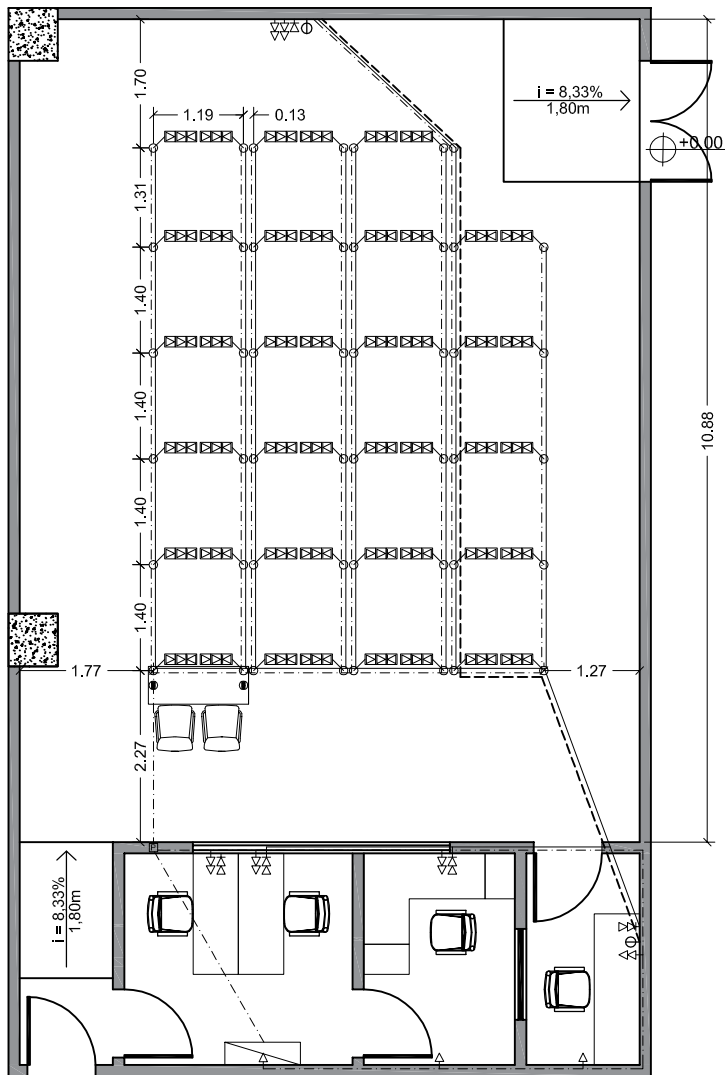
PROJETO ELÉTRICO PISO Escala 1/100
